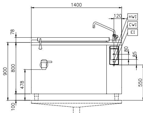
Front aanzicht
